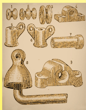
1885 Porcelain electrical insulators (La physique moderne : l'électricité dans la maison, É. Hospitalier)
